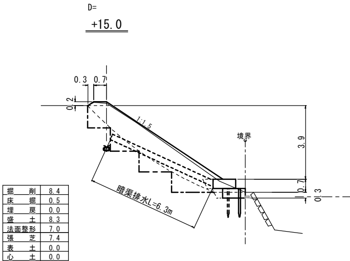
横断面図
