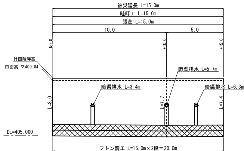
展開図 S=1:100
